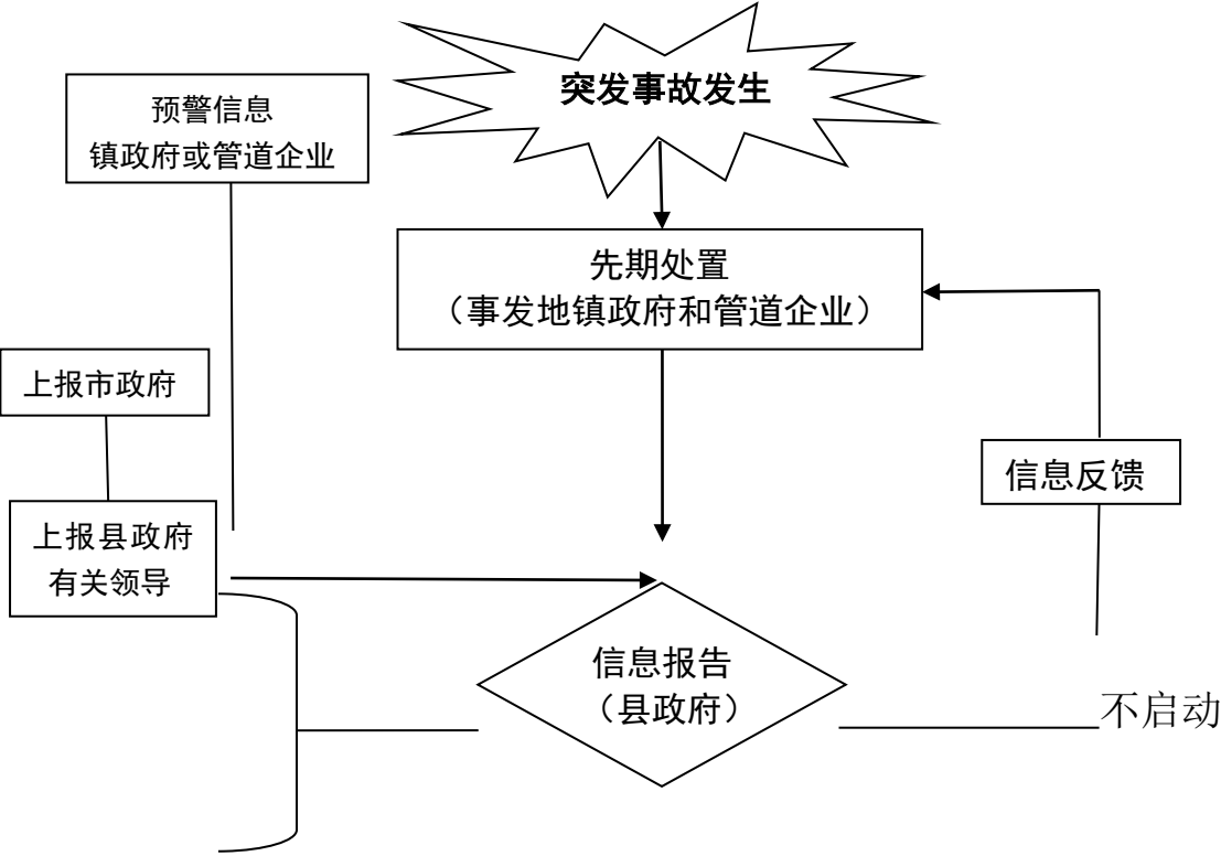
石油天然气管道突发事故应急处置流程
