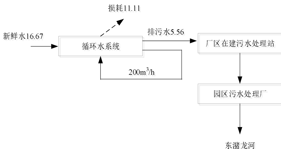
图 2-1a 拟建项目水平衡图 单位：m 3 /d
